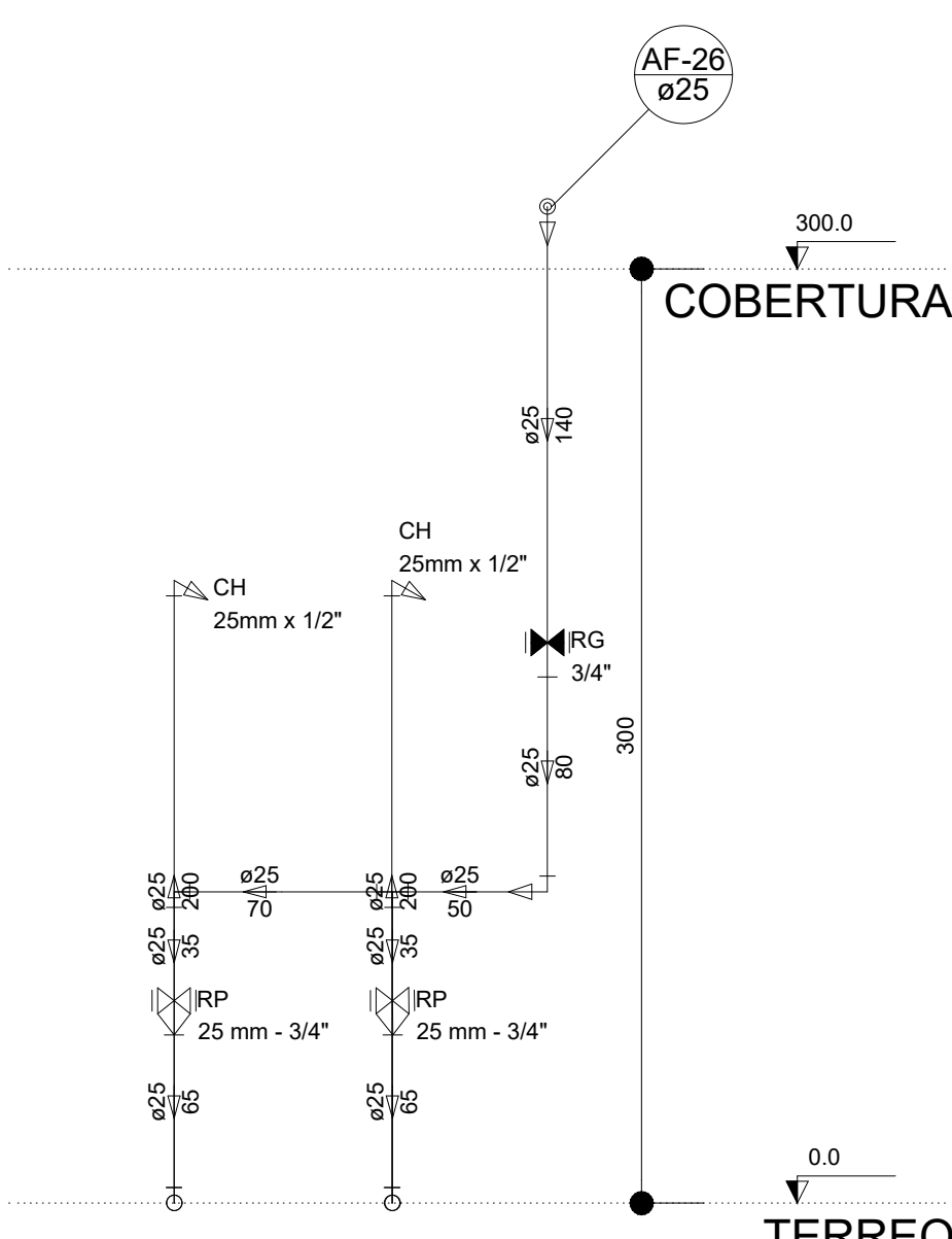
Corte C18 escala 1:25
