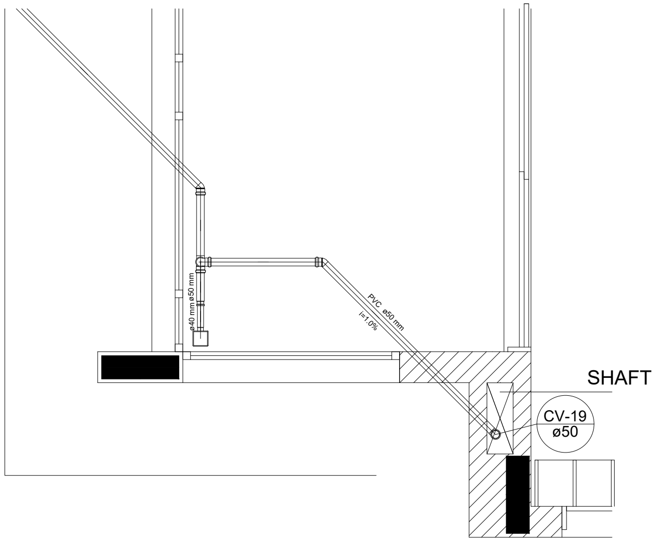
Detalhe S13 escala 1:25
