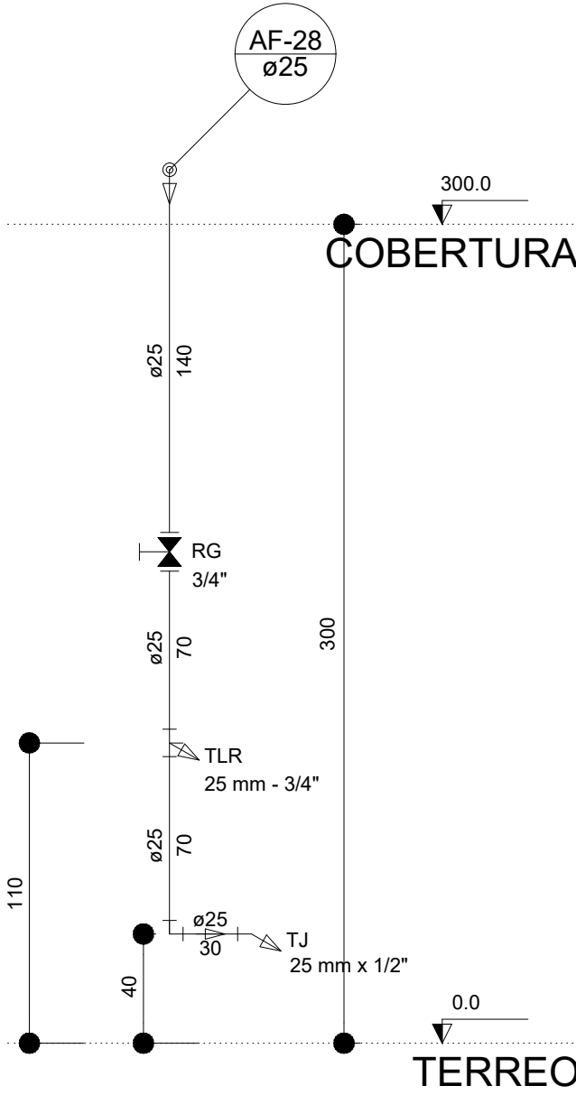
Corte C20 escala 1:25
