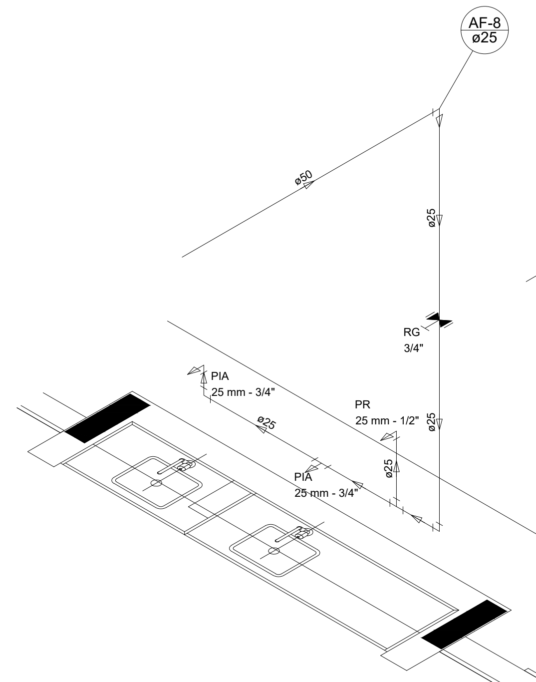
Detalhe H7 escala 1:25
