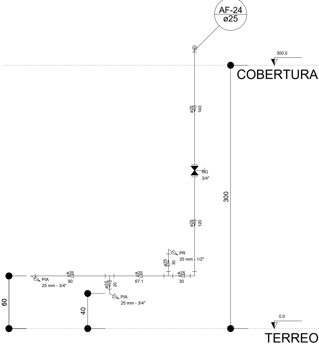
Corte C23 escala 1:25
