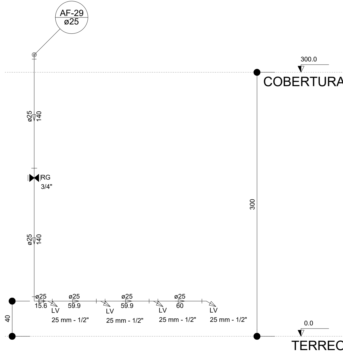
Corte C21 escala 1:25
