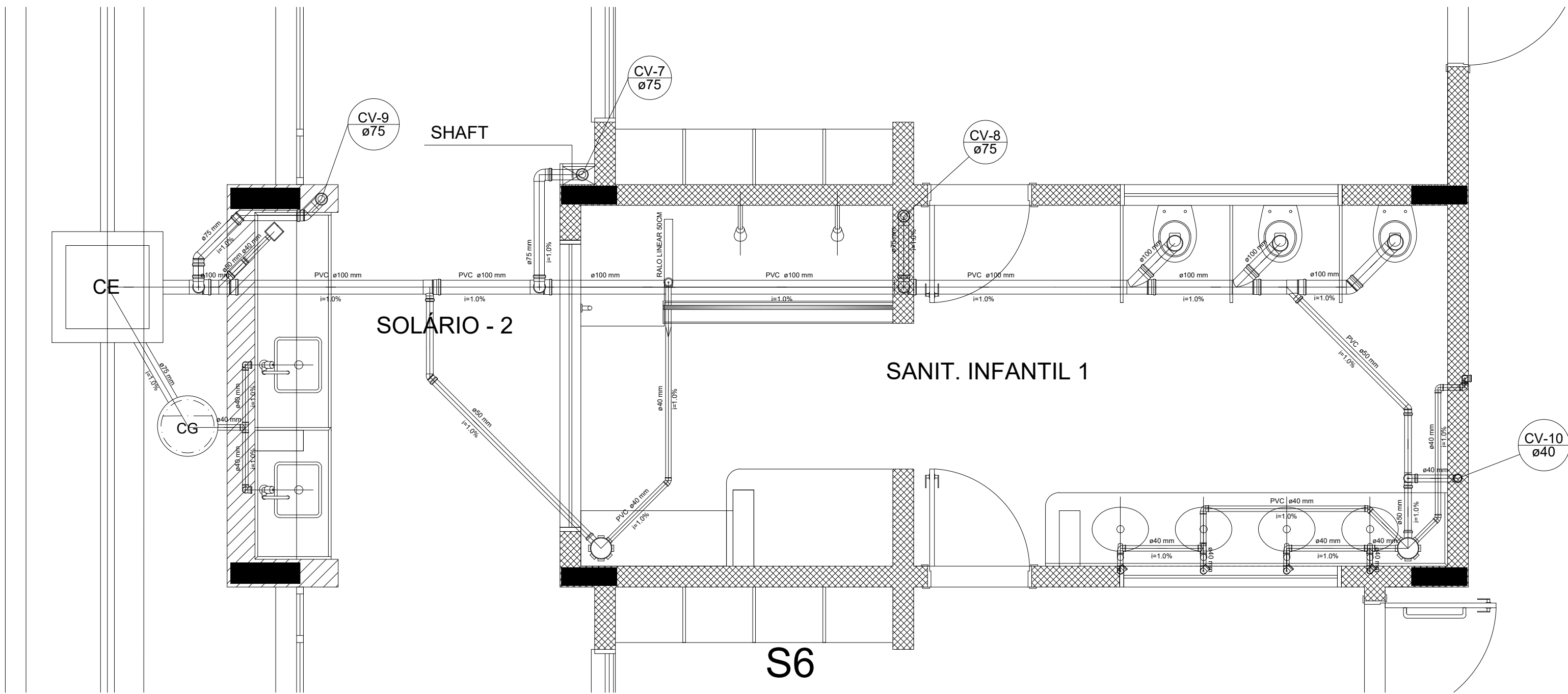
Detalhe S6 escala 1:25
