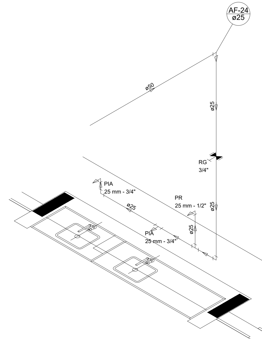
Detalhe H20 escala 1:25
