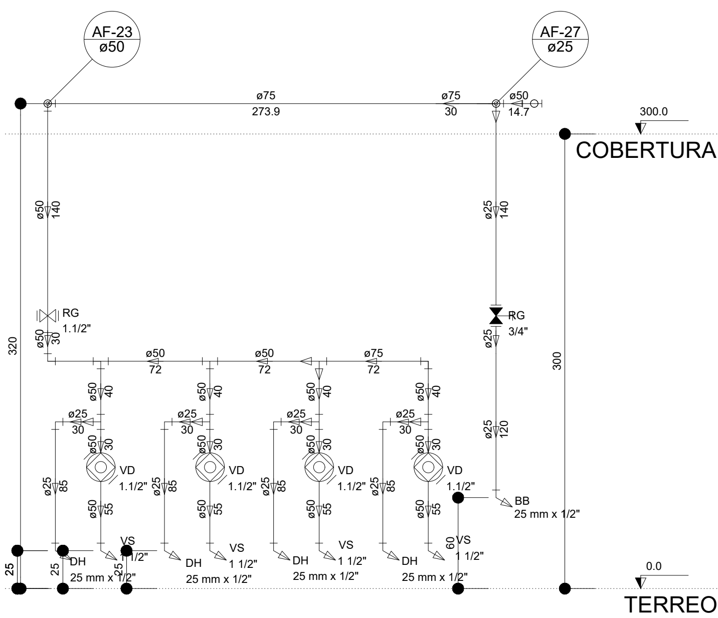
Corte C19 escala 1:25
