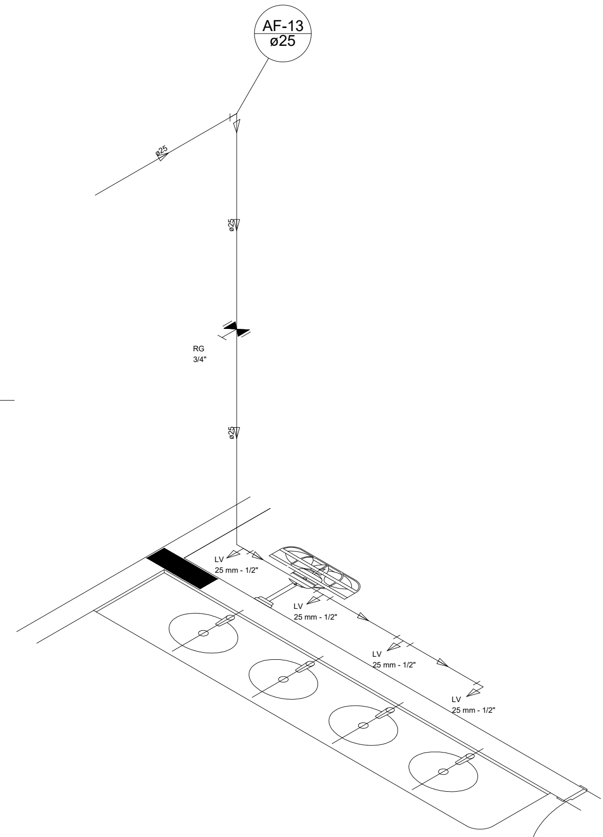
Detalhe H11 escala 1:25
