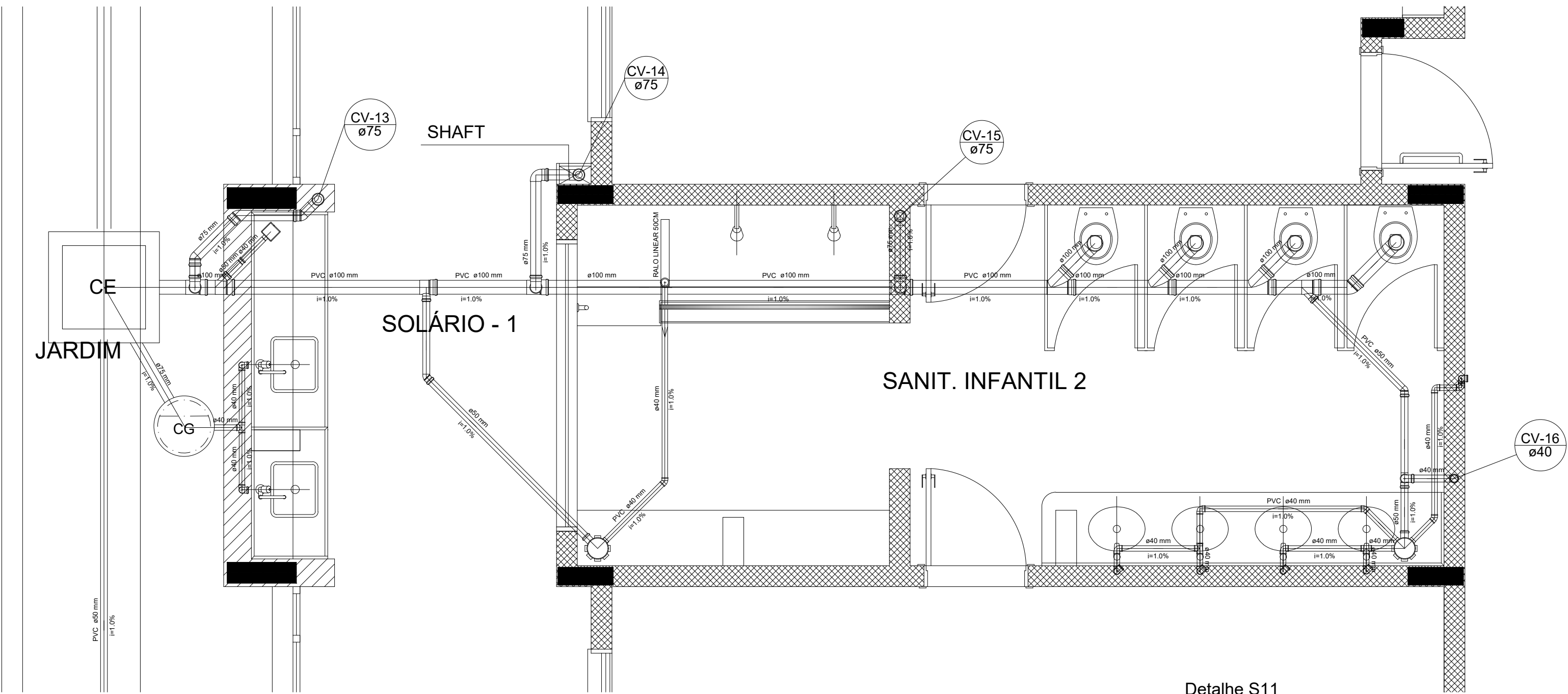
Detalhe S11 escala 1:25
