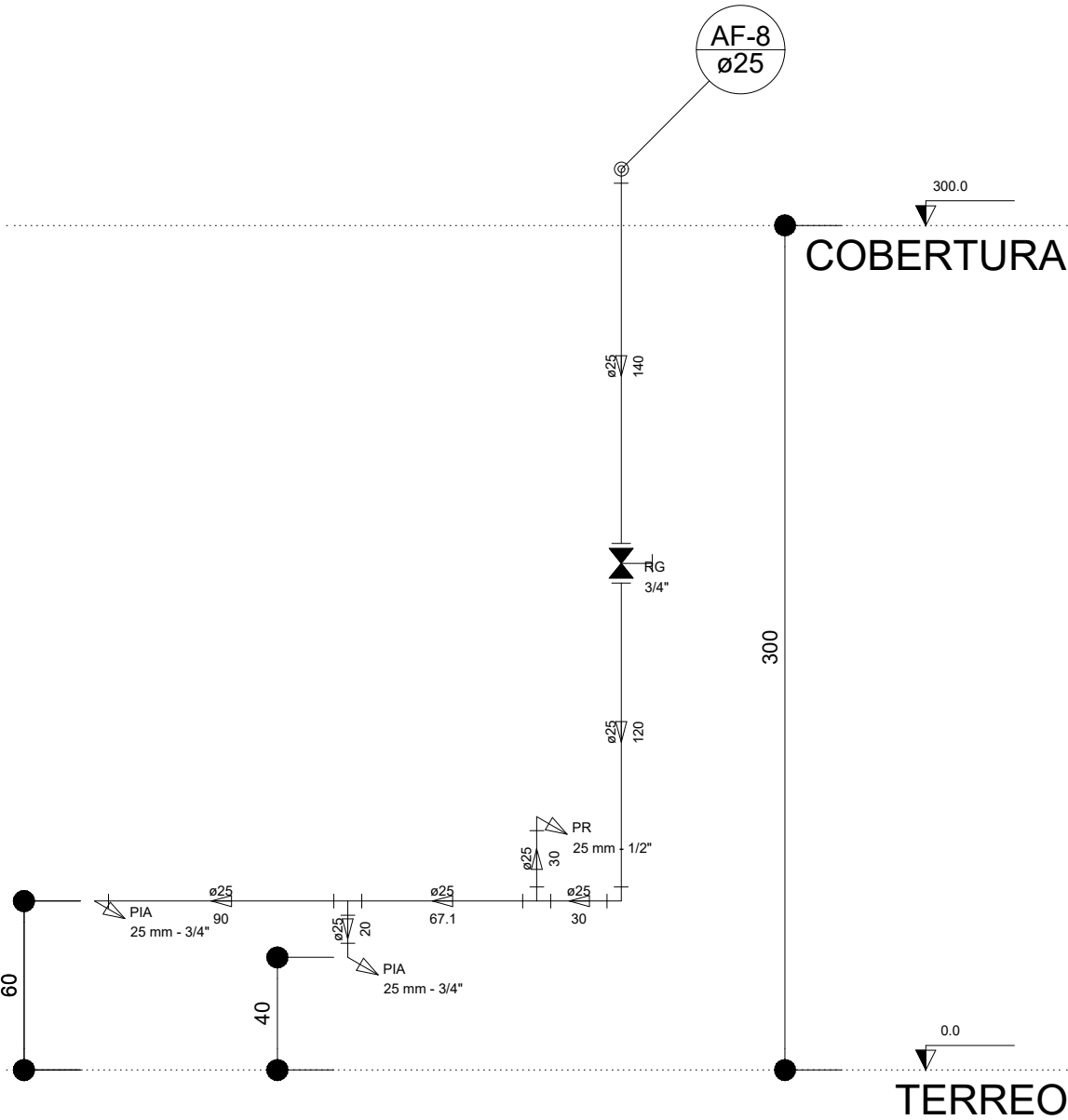
Corte C11 escala 1:25
