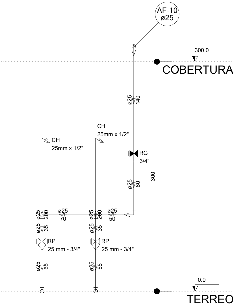
Corte C7 escala 1:25
