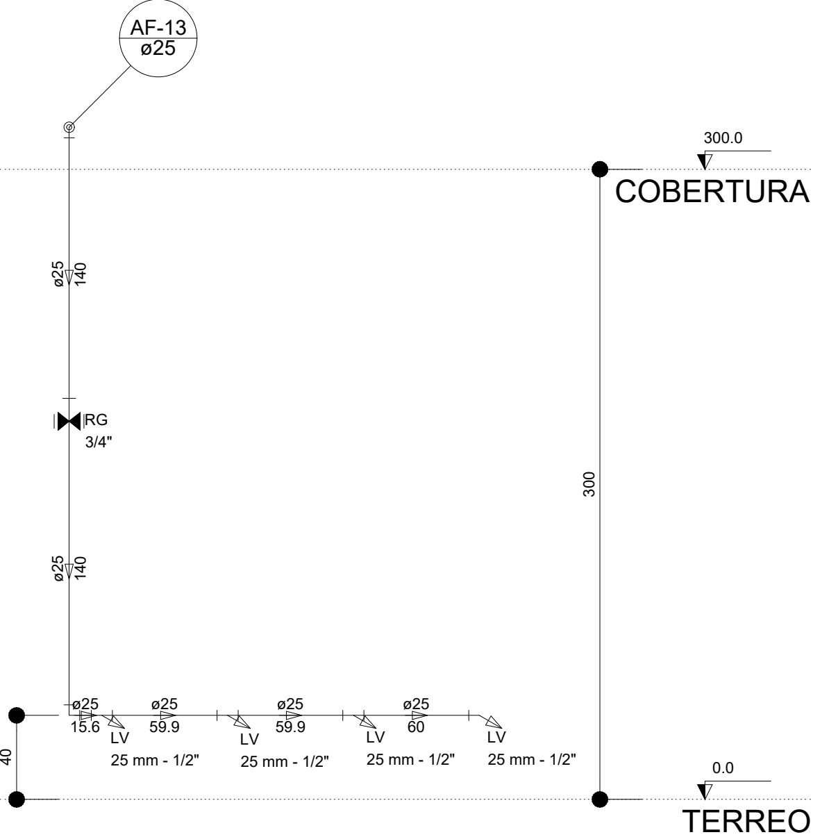
Corte C9 escala 1:25
