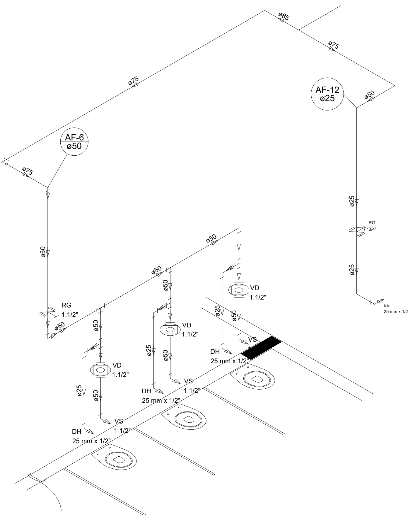
Detalhe H8 escala 1:25
