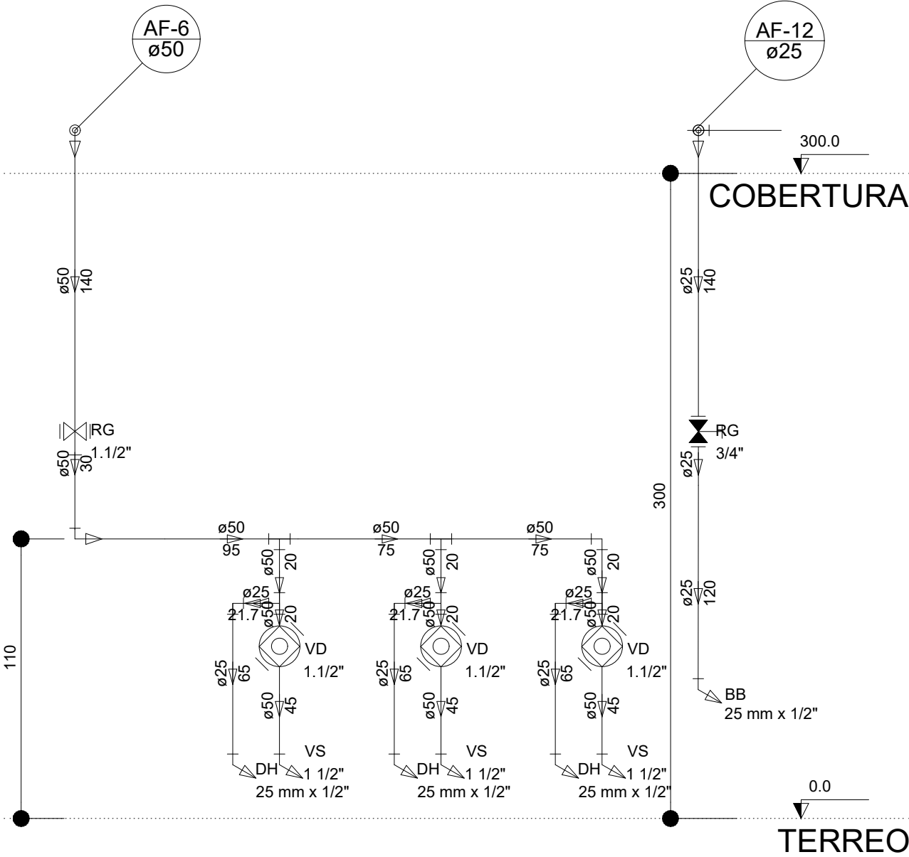
Corte C8 escala 1:25
