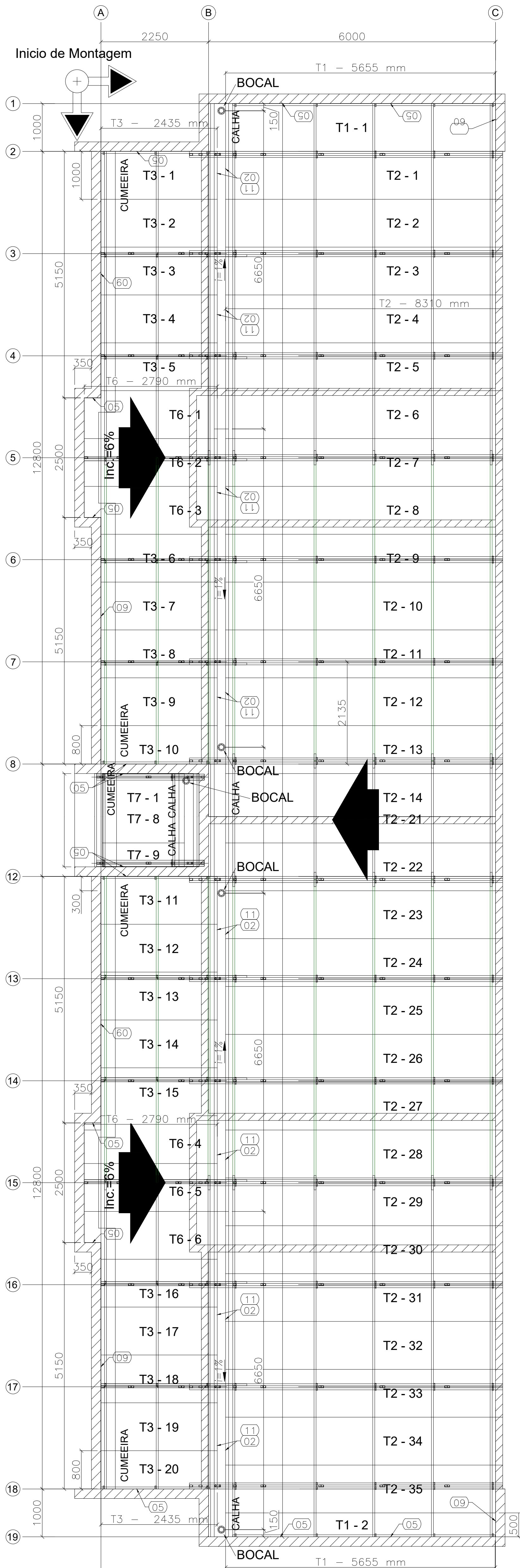
PLANTA DE COBERTURA
